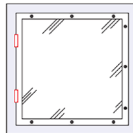
SVMK scharnierend en vast met schroeven
